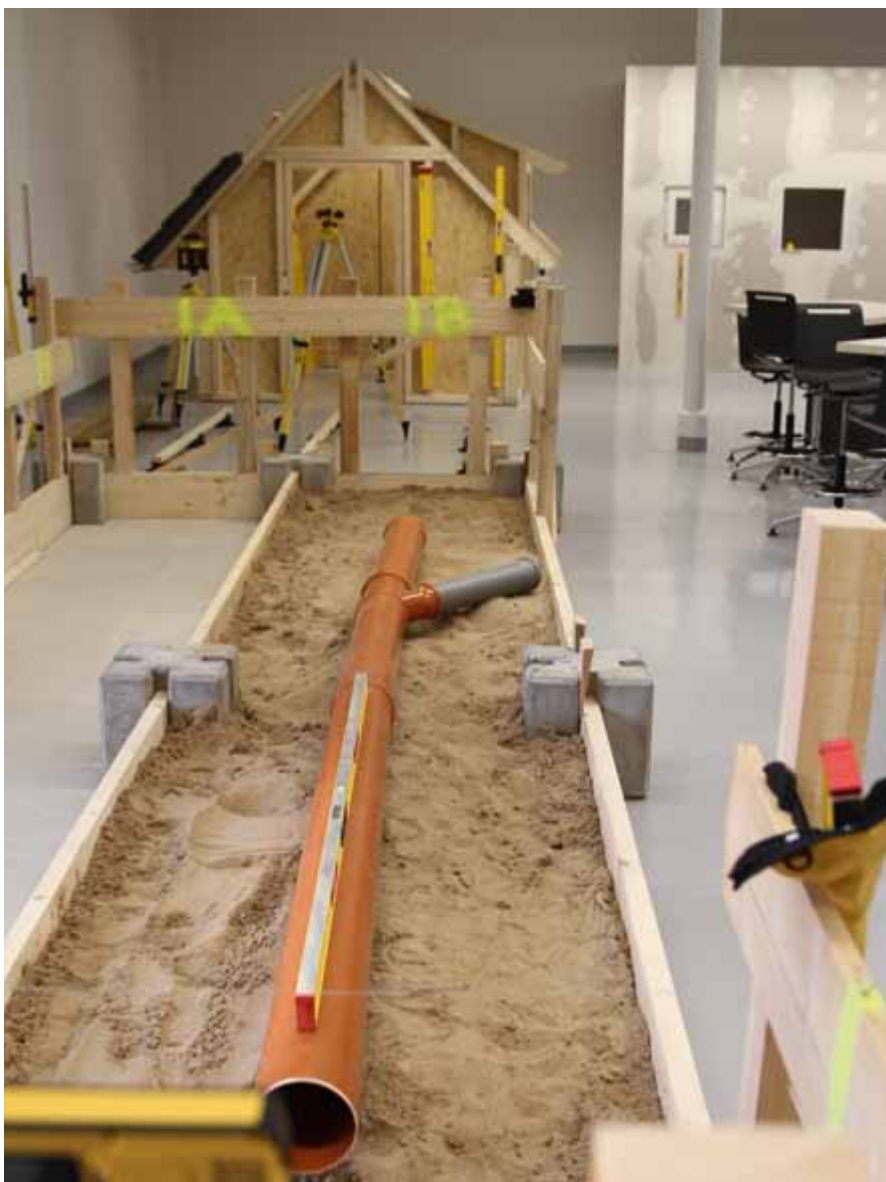
Zur Veranschaulichung von Messarbeiten im Tiefbau (z. B. Achsen übertragen, Wände anzeichnen oder Gefälle anlegen) wurde der „Sandkasten“ konzipiert. Am und im Holzhaus lassen sich typische Arbeiten des Zimmerers demonstrieren: rechte Winkel anlegen, Winkel und Innenmaße messen.
